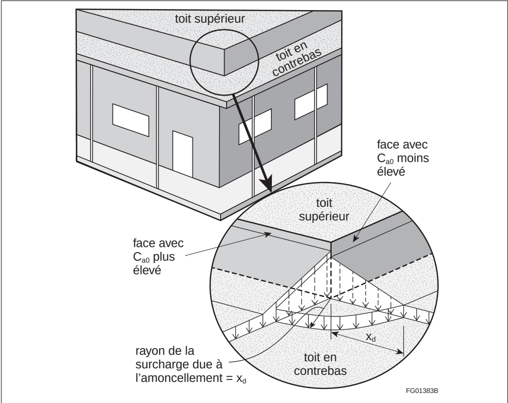
Figure 4.1.6.8.-A Charge due à la neige au coin extérieur Faisant partie intégrante du paragraphe 4.1.6.8. 1)
