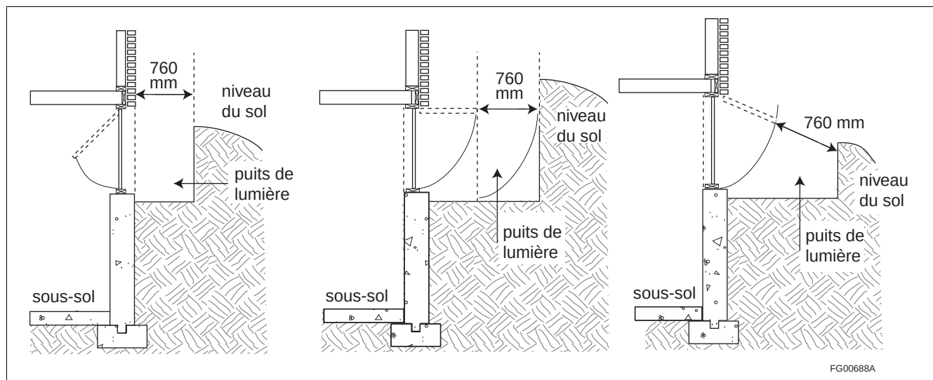
Figure A-9.9.10.1. 3) Fenêtre procurant un moyen d'évacuation ouvrant sur un puits de lumière
